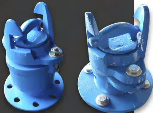
Extremo bridado para adaptar Cabeza Hidrante a Resorte/Bola
